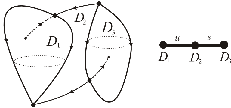
Fig. 1. Example of a flow and its bi-color graph Рис. 1. Пример потока и его двухцветного графа
