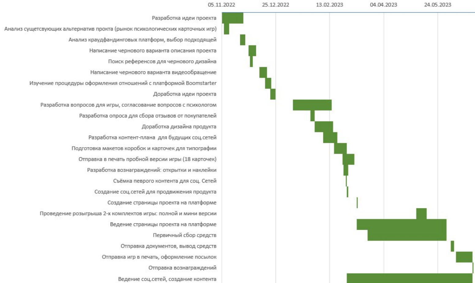
Диаграмма Ганта
