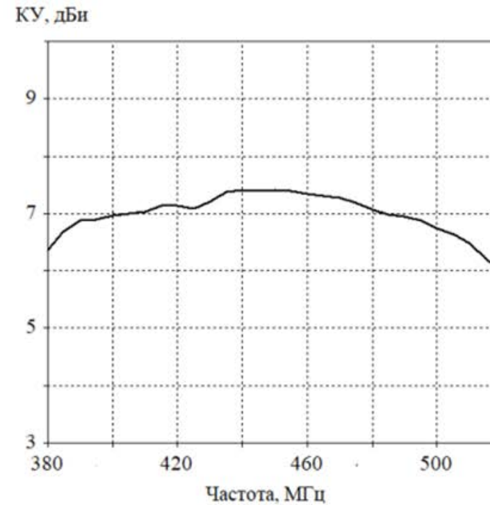
Рис. 2. Результаты моделирования: а) КСВ, б) КУ в направлении максимума излучения
