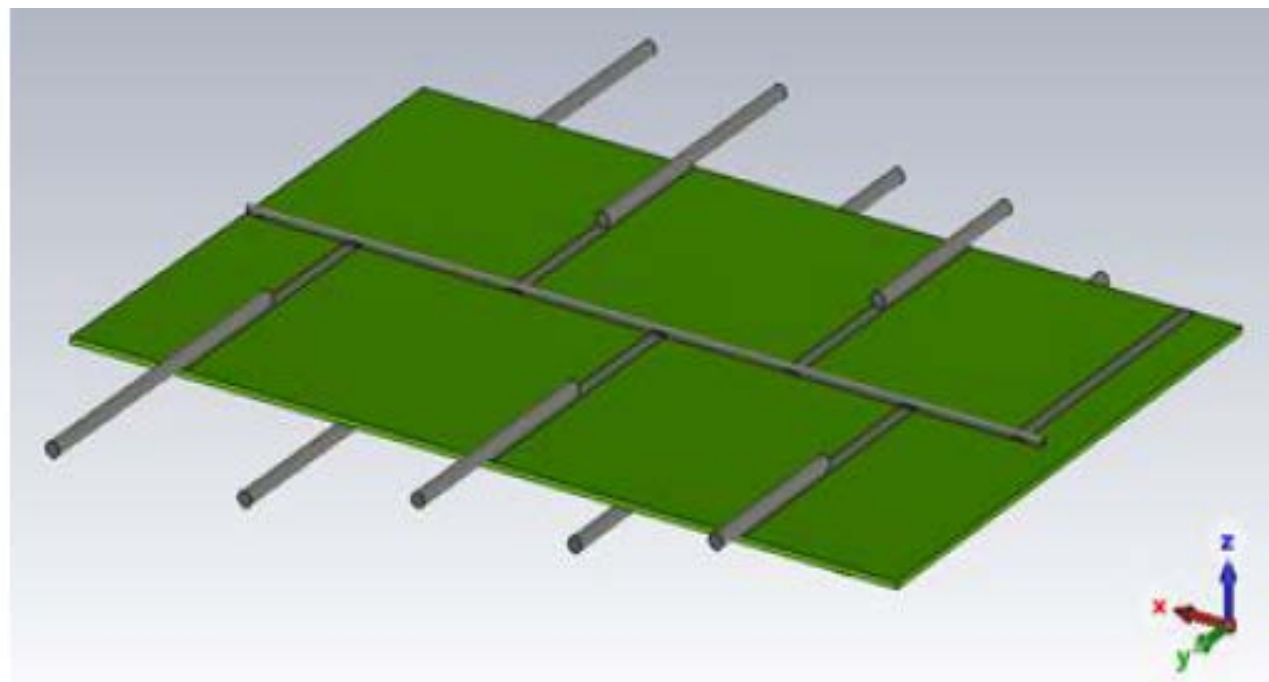
Рис. 1. Общий вид предложенной ЛПА.
