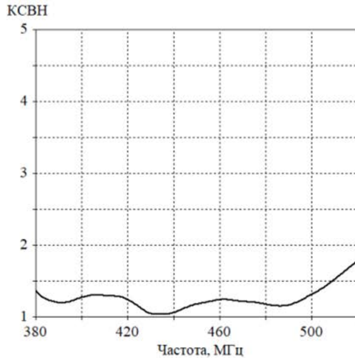
Рис. 2. Результаты моделирования: а) КСВ, б) КУ в направлении максимума излучения
